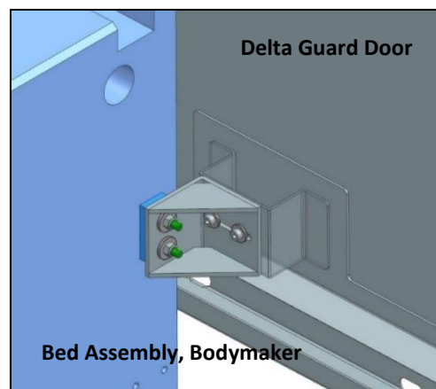
Fig. 2 - Neodymium Magnet Door Catch Assembly
