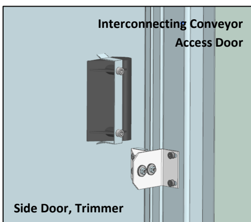
Fig. 3 - Neodymium Magnet Door Catch Assembly
